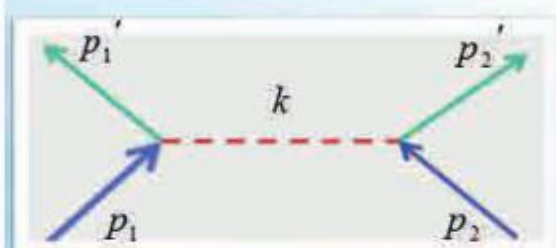
Рис. 2 Рассеяние электрона на электроне с обменом виртуальным фотоном
