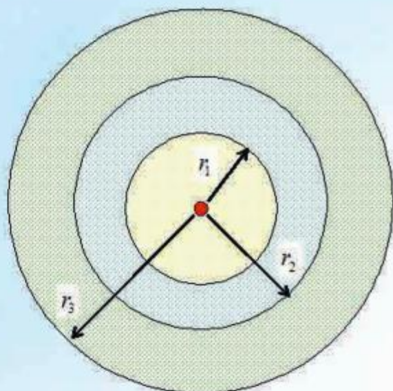
Рис.3 Модель элементарной частицы. r_i = \eta/m_i c, \quad i = 1, 2, 3.
